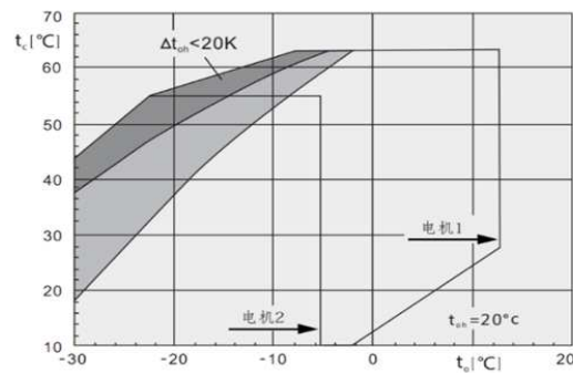
R22 Охлаждение всасывающим паром BS-SH-4H10-34÷BS-SH-6H50-151; BS-SH-4L8-41÷BS-SH-6L40-151
